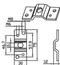
60.004.005 SOPORTE DE OBRA METAL 45MM. ESTRELLA
