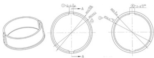
60.005.199 ADAPTADOR 55MM A 59MM
