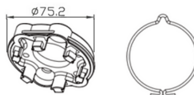
60.004.109 SOPORTE METÁLICO 45 BD + BDP+ WI
